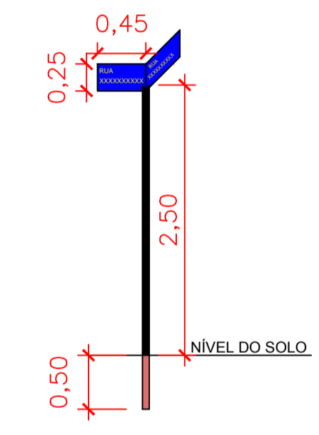
DET. PLACA LOGRADOURO ESCALA 1:50
