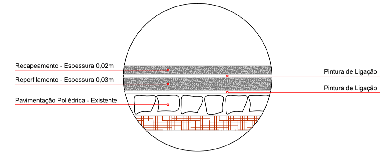
DET. CORTE TRANSVERSAL SEM ESCALA
