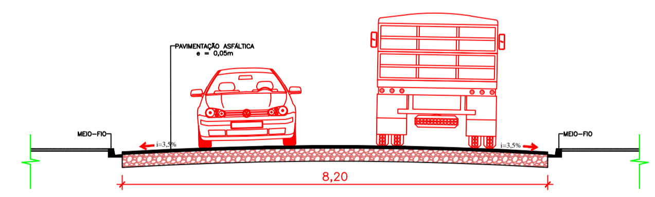
CORTE TRANSVERSAL ESCALA - 1:75
