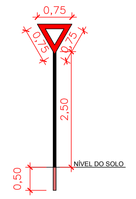
DET. PLACA R-02 ESCALA 1:50
