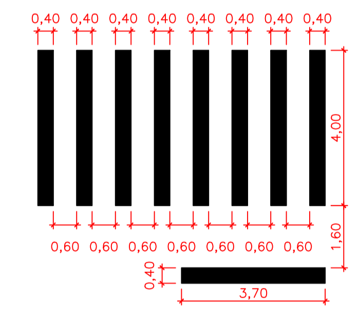
DET. FAIXA DE PEDRESTE ESCALA - 1:75
